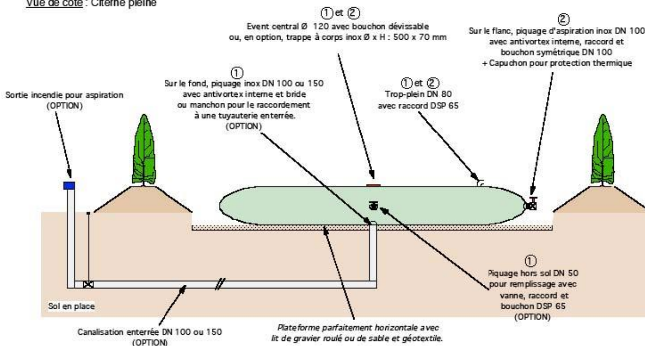
Vue de côté : Citerne pleine
